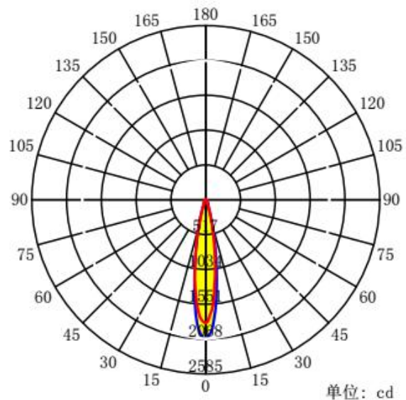
配光曲线
